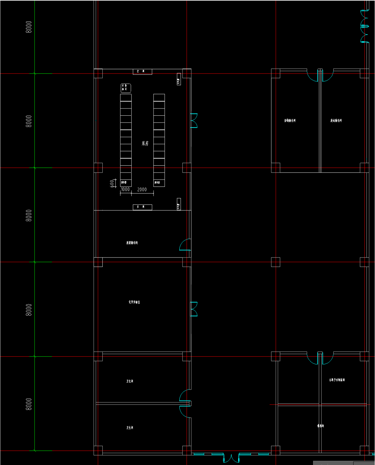
包头实验室 A 区布局图：
